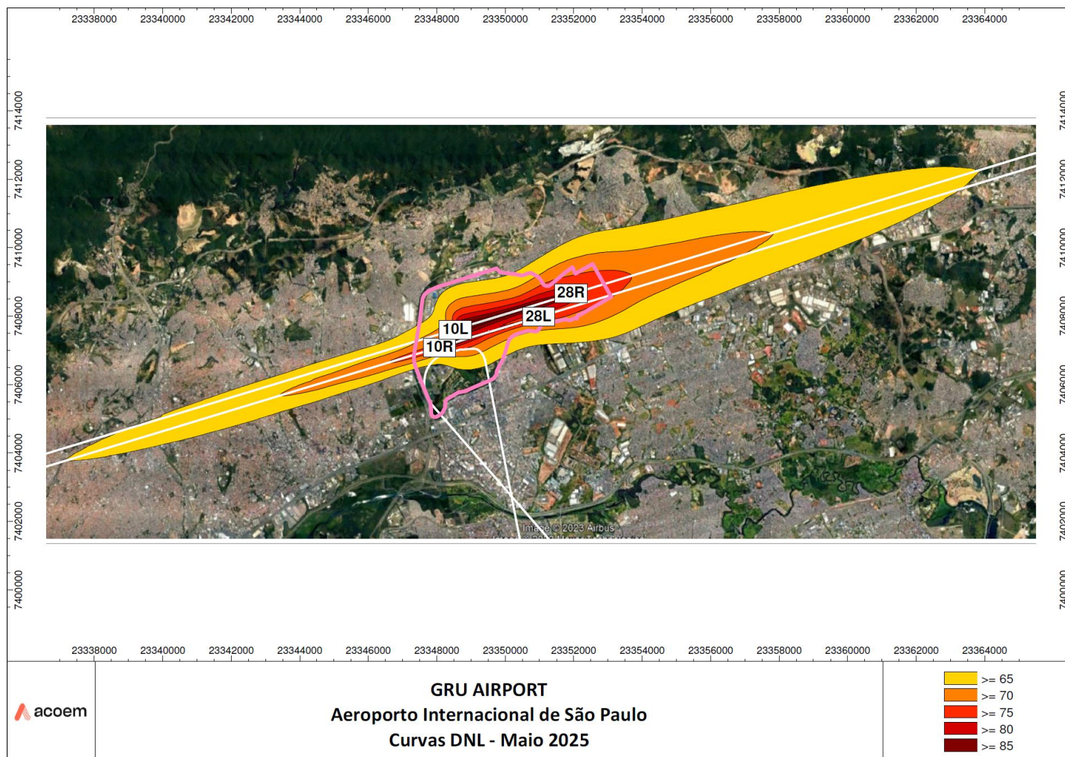
Figura 13 – Curvas de ruído DNL conforme RBAC nº161 com imagens de satélite – Maio/2025.
