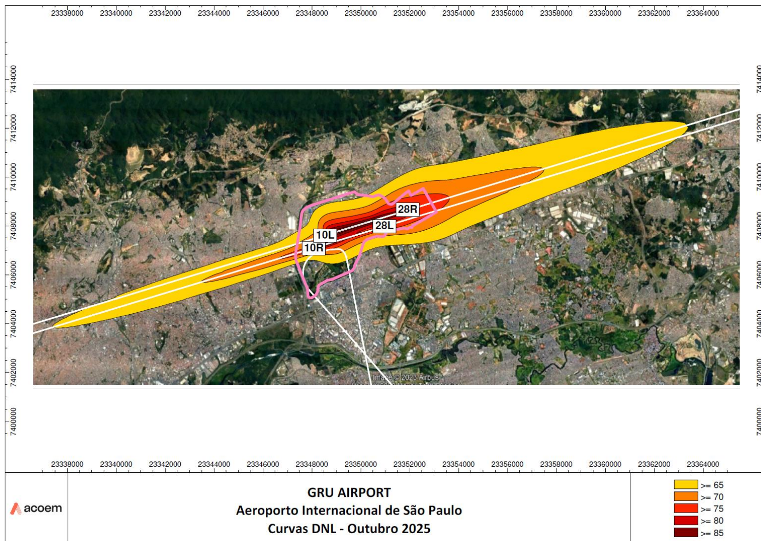
Figura 18 – Curvas de ruído DNL conforme RBAC n°161 com imagens de satélite – Outubro/2025.
