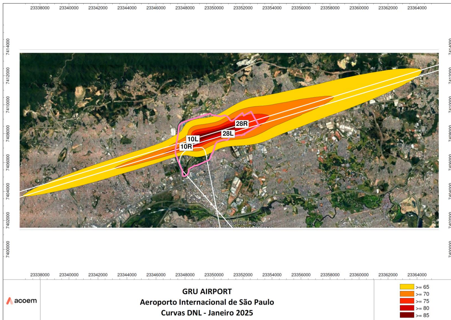
Figura 9 – Curvas de ruído DNL conforme RBAC n°161 com imagens de satélite – Janeiro/2025.
