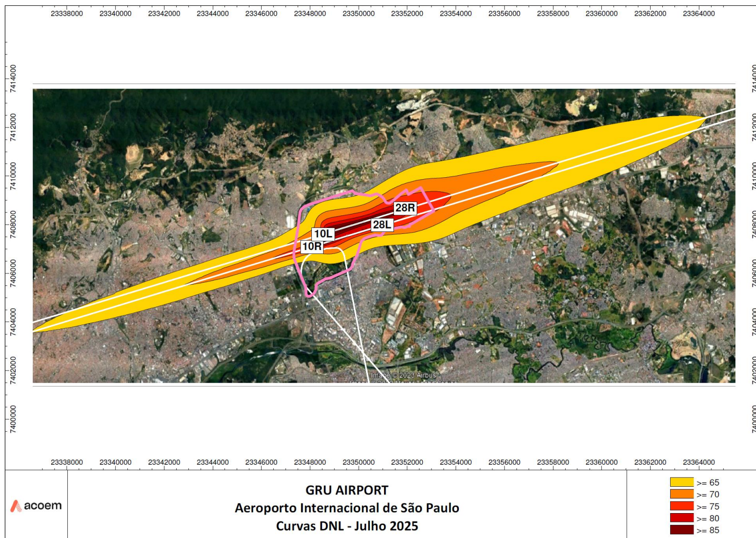
Figura 15 – Curvas de ruído DNL conforme RBAC n°161 com imagens de satélite – Julho/2025.
