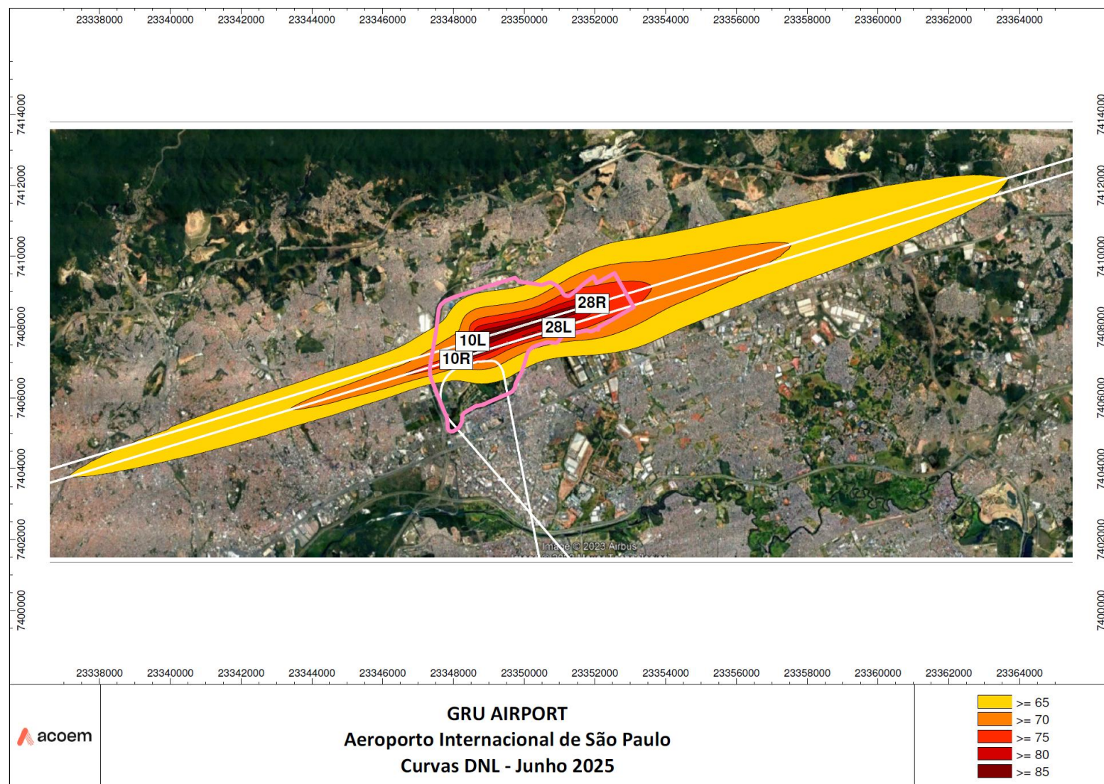
Figura 14 – Curvas de ruído DNL conforme RBAC n°161 com imagens de satélite – Junho/2025.
